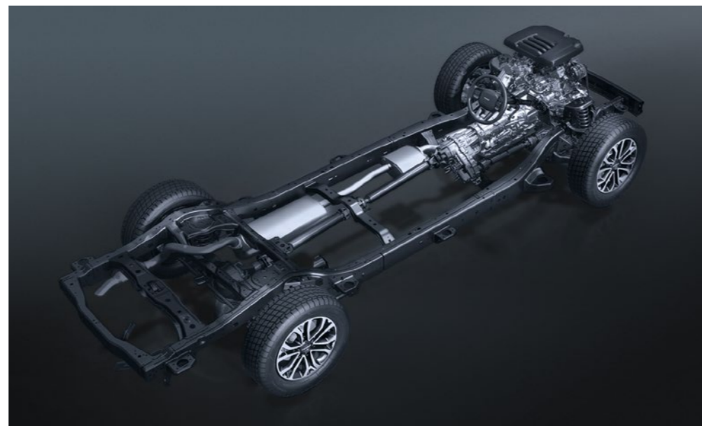
Рамная конструкция кузова
